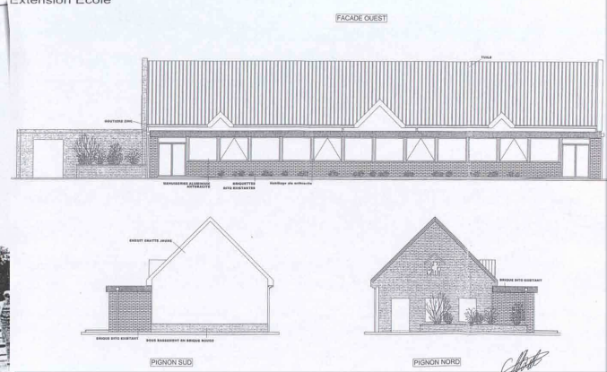
MAIRIE DE NORTKERQUE Extension Ecole
